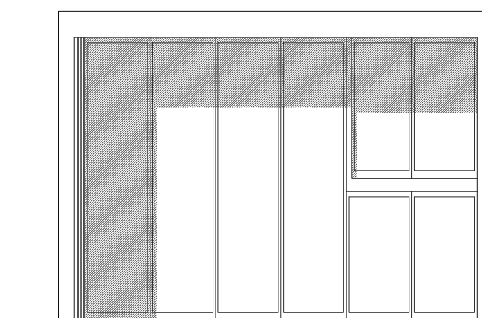
ALZADO FRONTAL (BRISE-SOLEIL RECOGIDOS)
