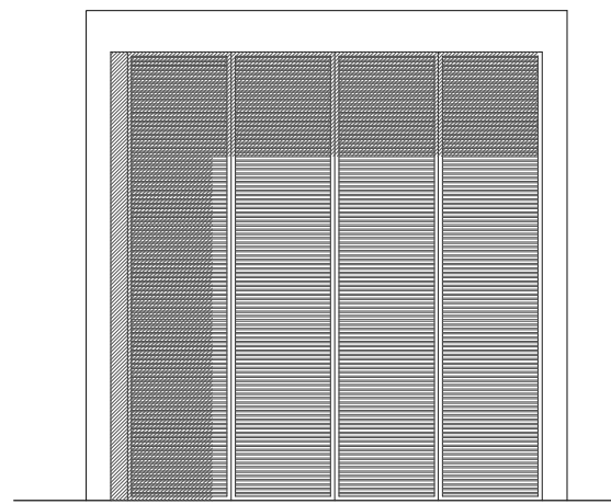
ALZADO FRONTAL (BRISE-SOLEIL EXTENDIDOS)
