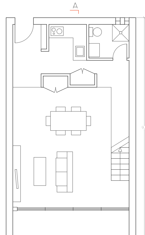
PLANTA BAJA
