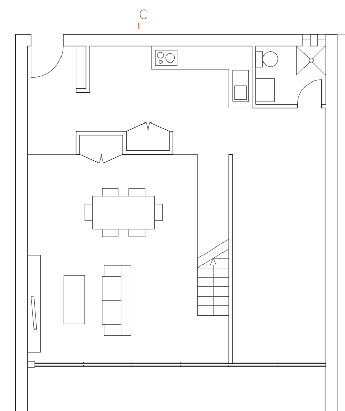
PLANTA BAJA
