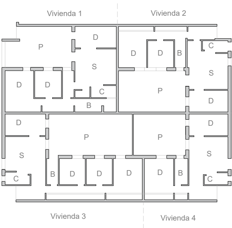
TIPOLOGÍA DE VIVIENDA E:1/200
